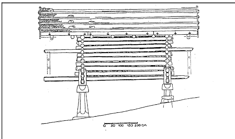
Fig. 6 - Lato est. Stipiti della porta e soglia ricostruita.
