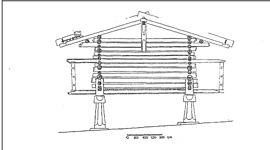
Fig. 1 - Sezione trasversale
