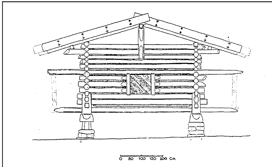
Fig. 6 - Lato est. Stipiti della porta e soglia ricostruita.
