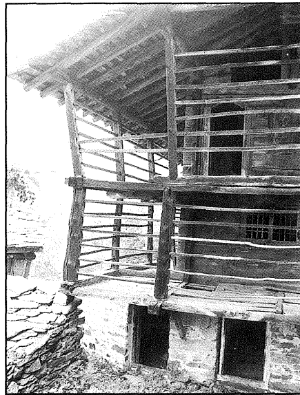
Alagna: loc. Wold: Loggiati a griglia e piano terreno in muratura.
